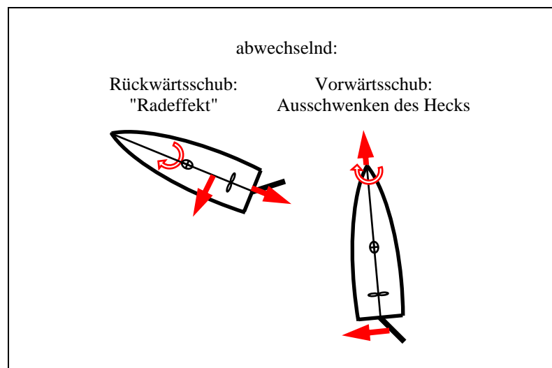
Abb. 3-5: "Drehen auf dem Teller"
