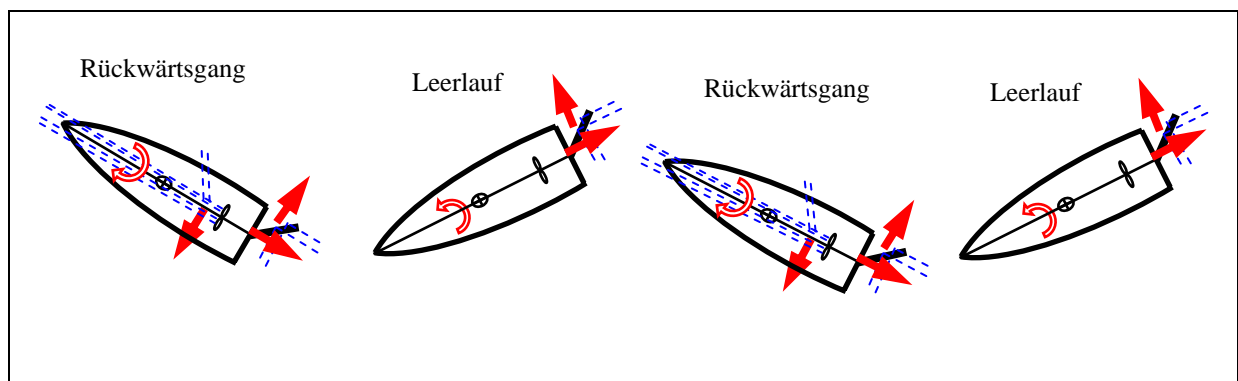
Abb. 3-4: Fahrt zurück mit starkem "Radeffekt" und Impuls-Schub
