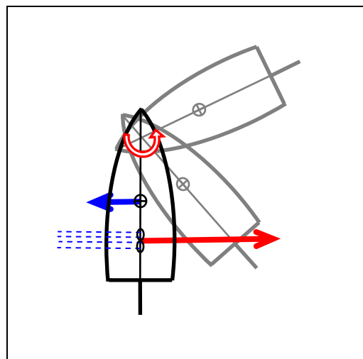
Abb. 3-10: Drehung eines drehbaren Antriebs bei 90^\circ Anstellwinkel
