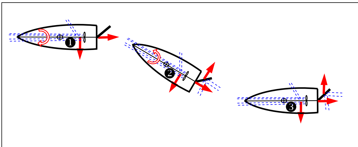
Abb. 3-3: Fahrt zurück unter Motor mit Radeffekt ("linksdrehender" Propeller)
