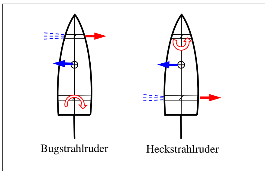
Abb. 3-7: Kräfte und Drehmomente von Bug- und Heckstrahlruder
