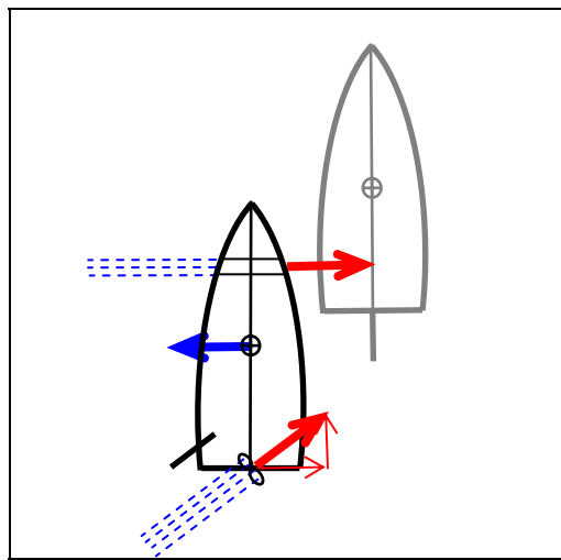
Abb. 3-11: Drehbarer Antrieb plus Bugstrahlruder
