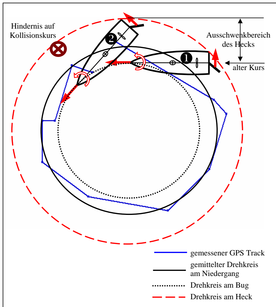
Abb. 3-2: Eigenschaften des Drehkreises vorwärts unter Motor
