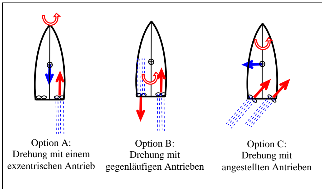
Abb. 3-12: Parallel drehbare Doppelantriebe: Drehbewegungen
