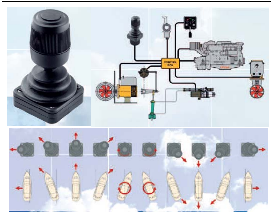
Abb. 5-4: Vetus Pro-Docker System (Quelle: Vetus)
