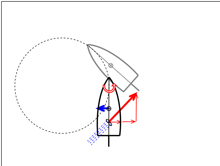
Abb. 3-9: Kräfte und Drehmomente eines drehbaren Antriebs
