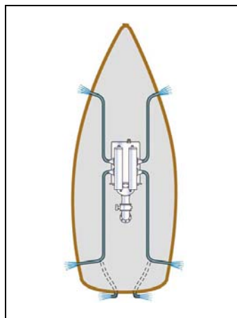
Abb. 3-14: Pumpjet für Wassersportfahrzeuge (Quelle: Broschüre der Fa. Willdo)
