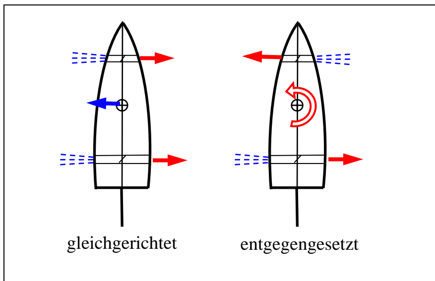
Abb. 3-8: Bug- und Heckstrahlruder im Verbund
