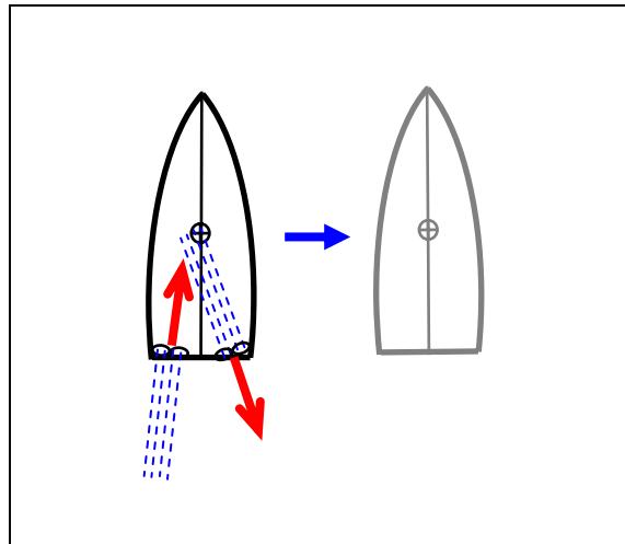
Abb. 3-13: Individuell ansteuerbare Doppelantriebe: Querschub
