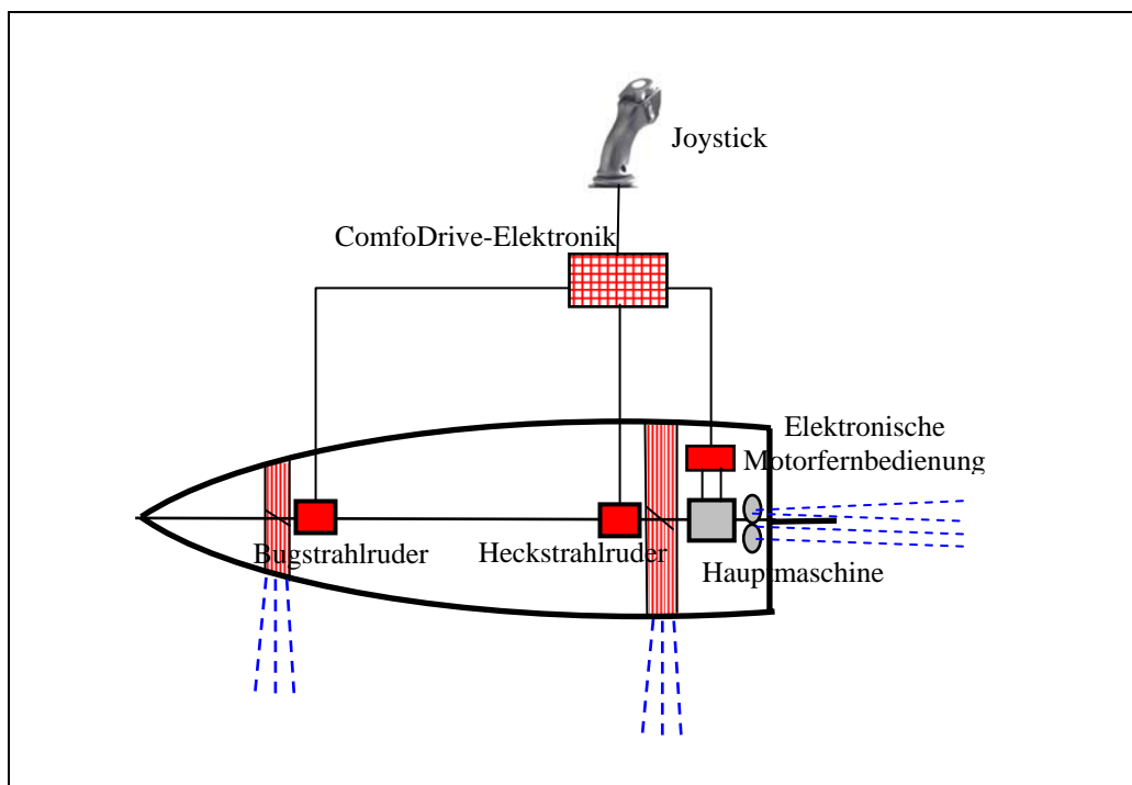
Abb. 5-1: Technisches ComfoDrive-Konzept
